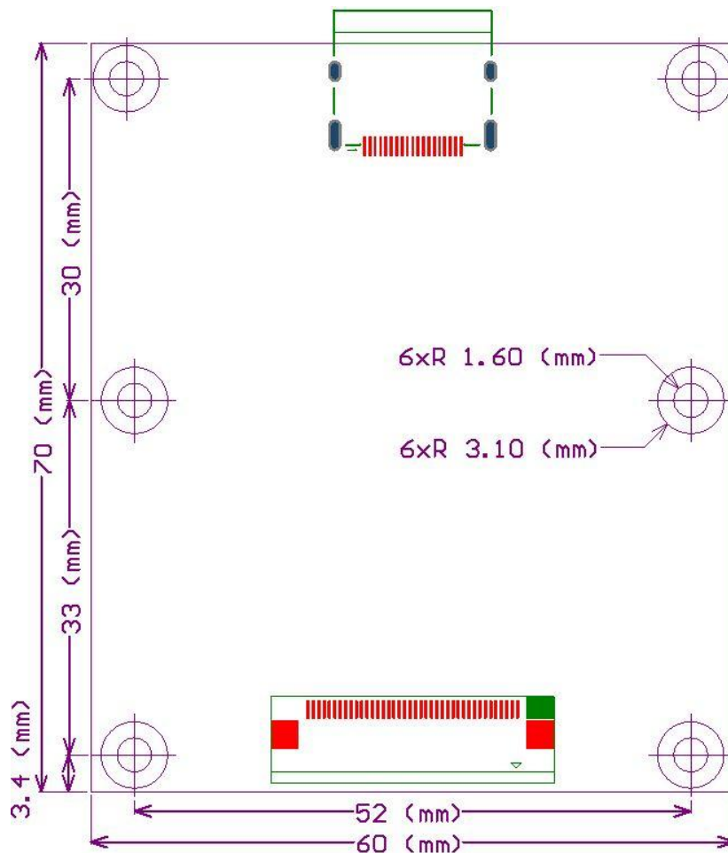
ETA924 外形尺寸（单位：mm）
