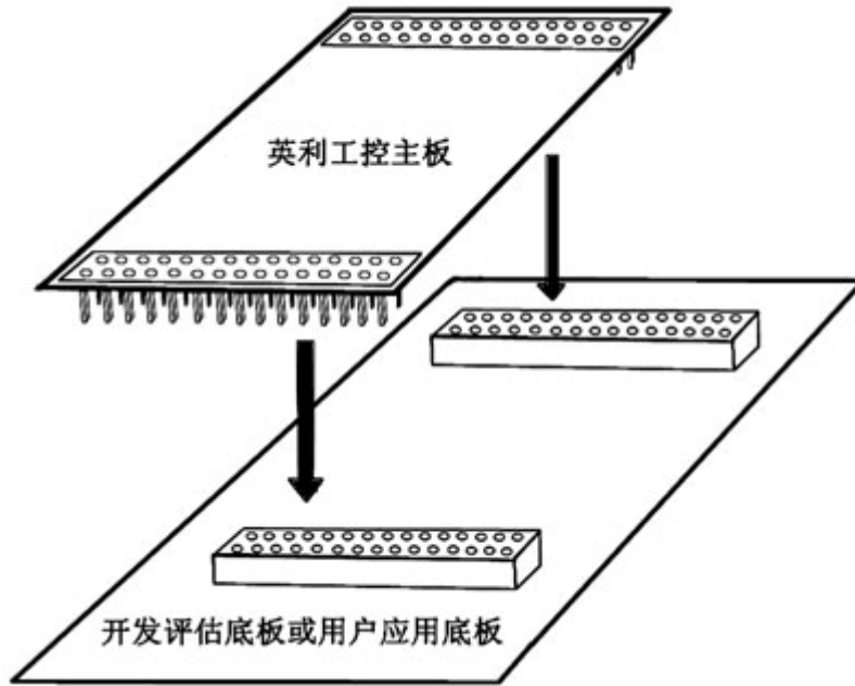
图 2_1: 英利工控主板与开发评估底板的连接关系
