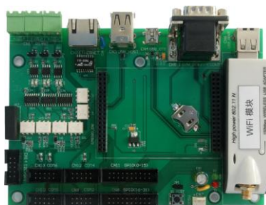
1 块与之对应的 EM9380 开发评估底板和 1 个 WiFi 模块
