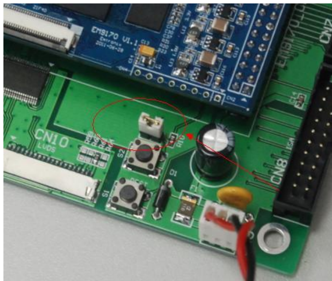
图 1-1 JP1，模式切换跳线器
